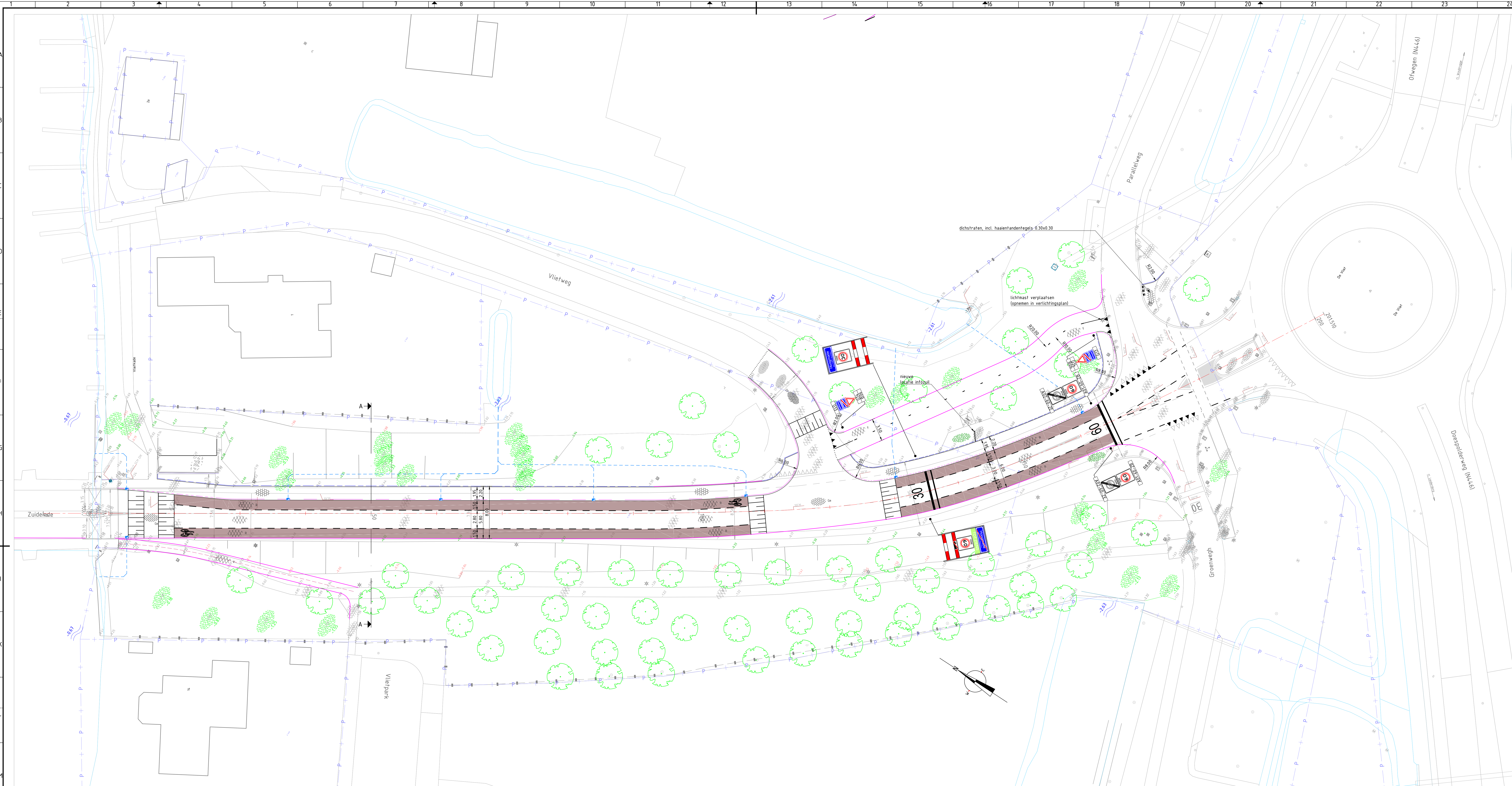
Situatie Zuidende Schaal 1:200
